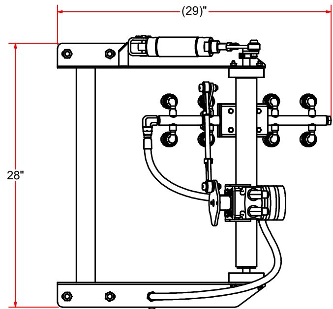
TOP
