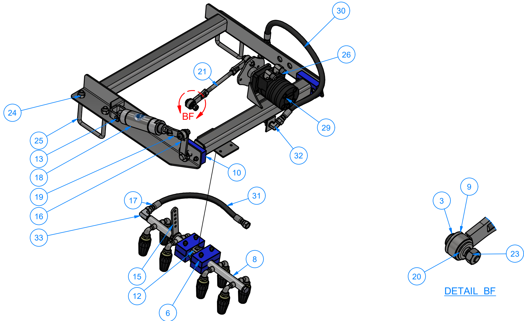
VIEW139
