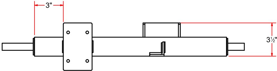
BOTTOM
