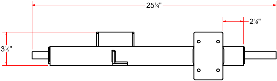
BOTTOM
