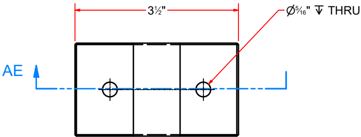
TOP
