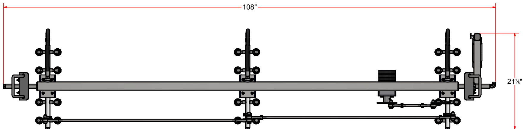
TOP
