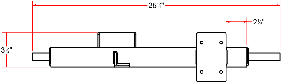
BOTTOM
