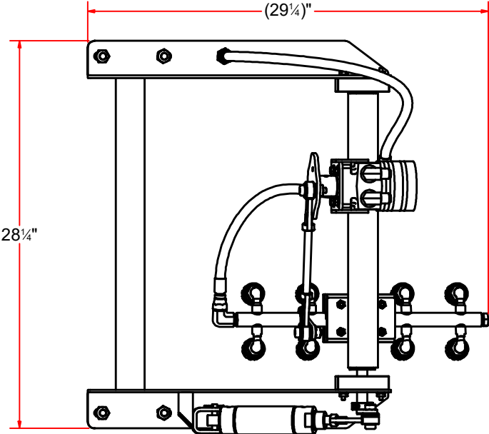
TOP
