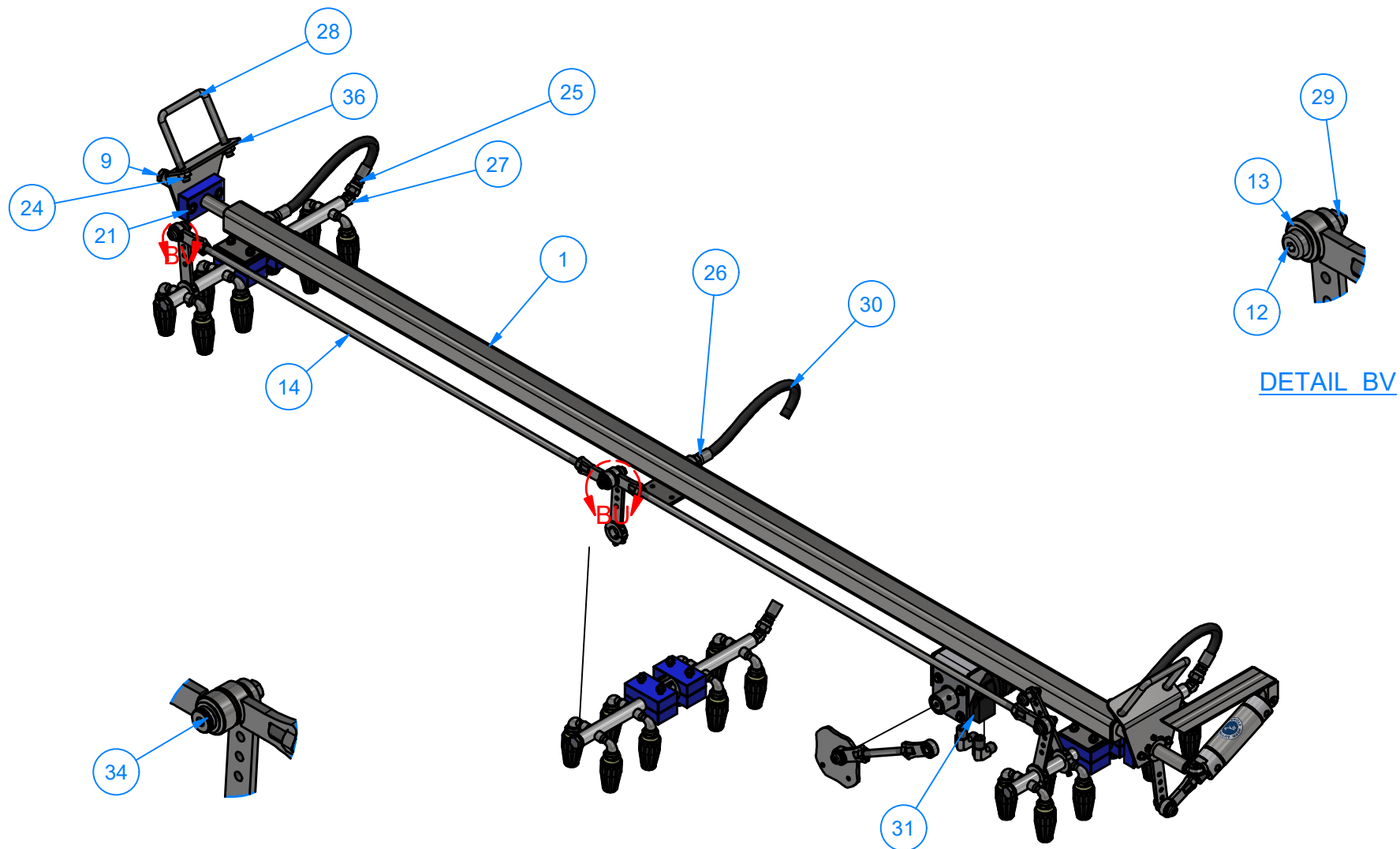
DETAIL BU
