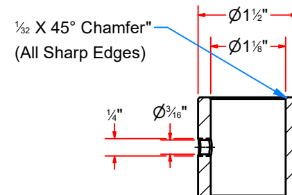
SECTION AK-AK
