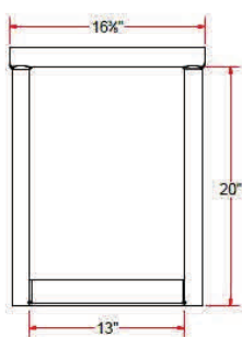
STAND DIMENSIONS
