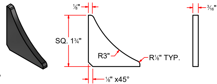
GUSSS187X0175X0175 - Gusset #7Ga x 1 3/4 x 1 3/4
