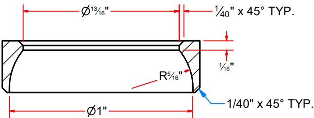
SECTION AB-AB SCALE 2 : 1
